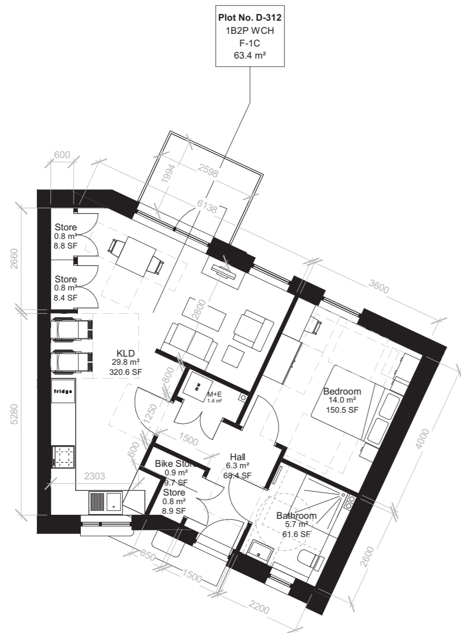
Flat Type F-1C (wch)
