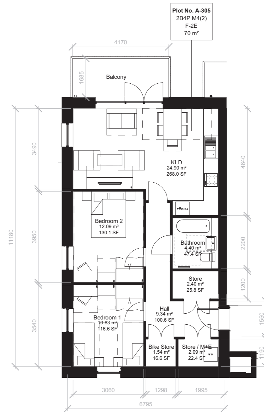
Flat Type F-2E
