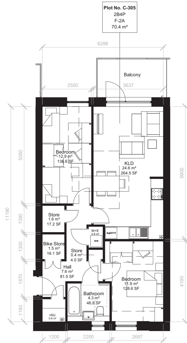
Flat Type F-2A
